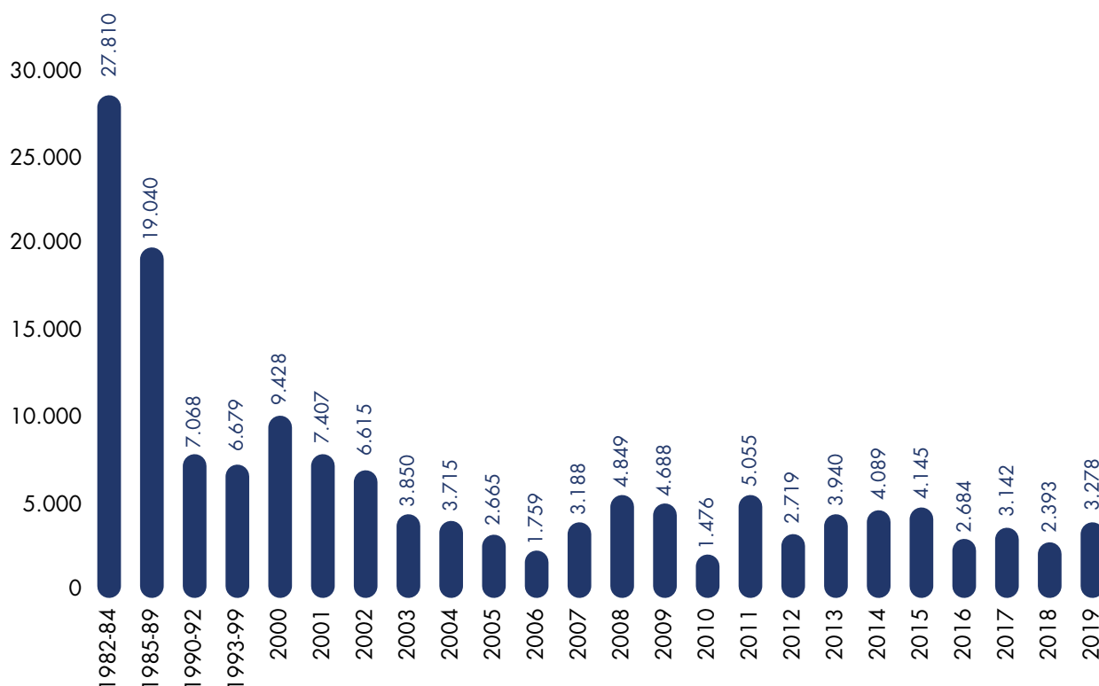
Grafico 6.15 FOSFORO RESIDUO RILASCIATO DAL DEPURATORE DI COMACCHIO - KG/ANNO
