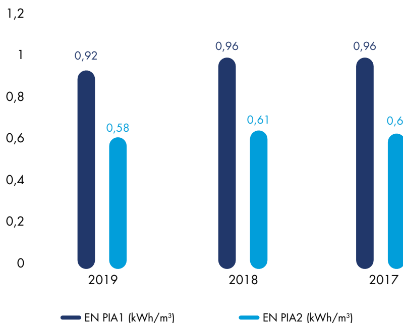
Grafico 6.18 INDICE D'INTENSITÀ ENERGETICA
